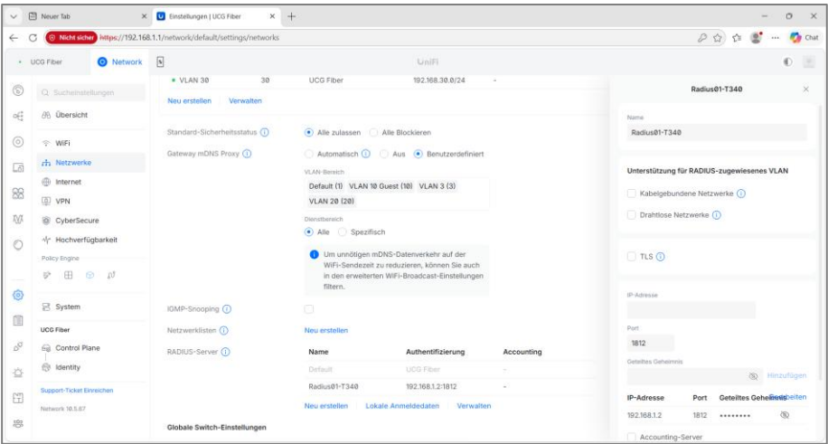
Radius-Server Konfiguration auf einem UniFi Cloud Gateway Fiber
