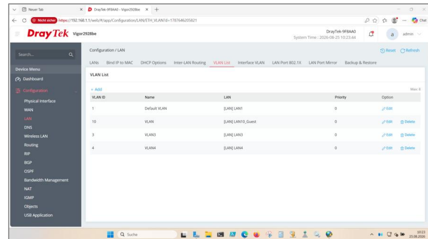
Configuration | LAN | VLAN List
