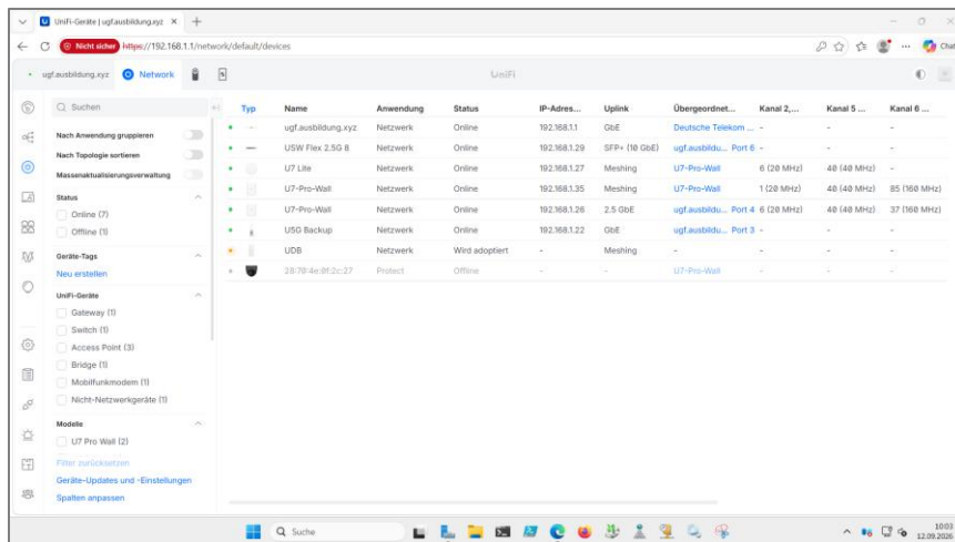
3) UGF Network | Devices: Die Device Bridge (UDB) wird adoptiert
